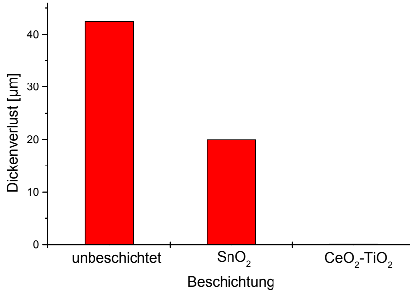
Bild 1: Schichtdickenverlust bzw. Glasverlust bei Alkaliangriff (30 gew.%ige NaOH, 1 d 90 °C) auf unbeschichtetes und beschichtetes Borosilicatglas.
