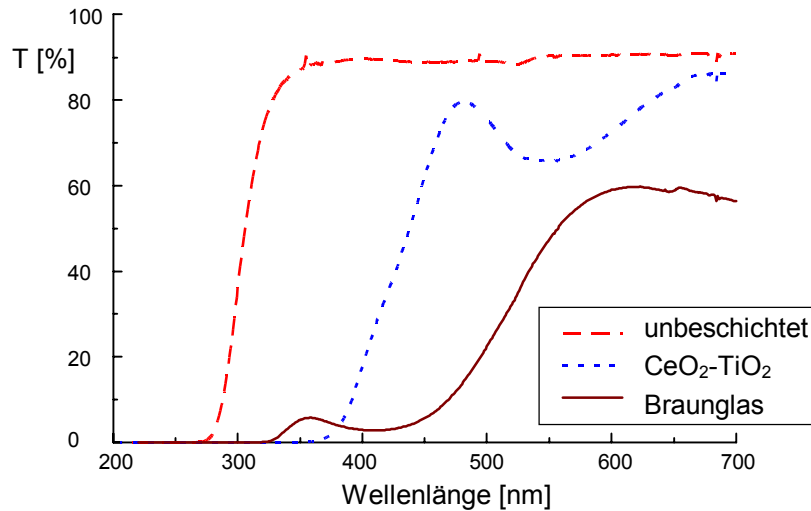
Bild 2: Transmissionsspektren von unbeschichtetem und CeO 2 -TiO 2 -beschichtetem Borosilicatglas sowie von Braunglas
